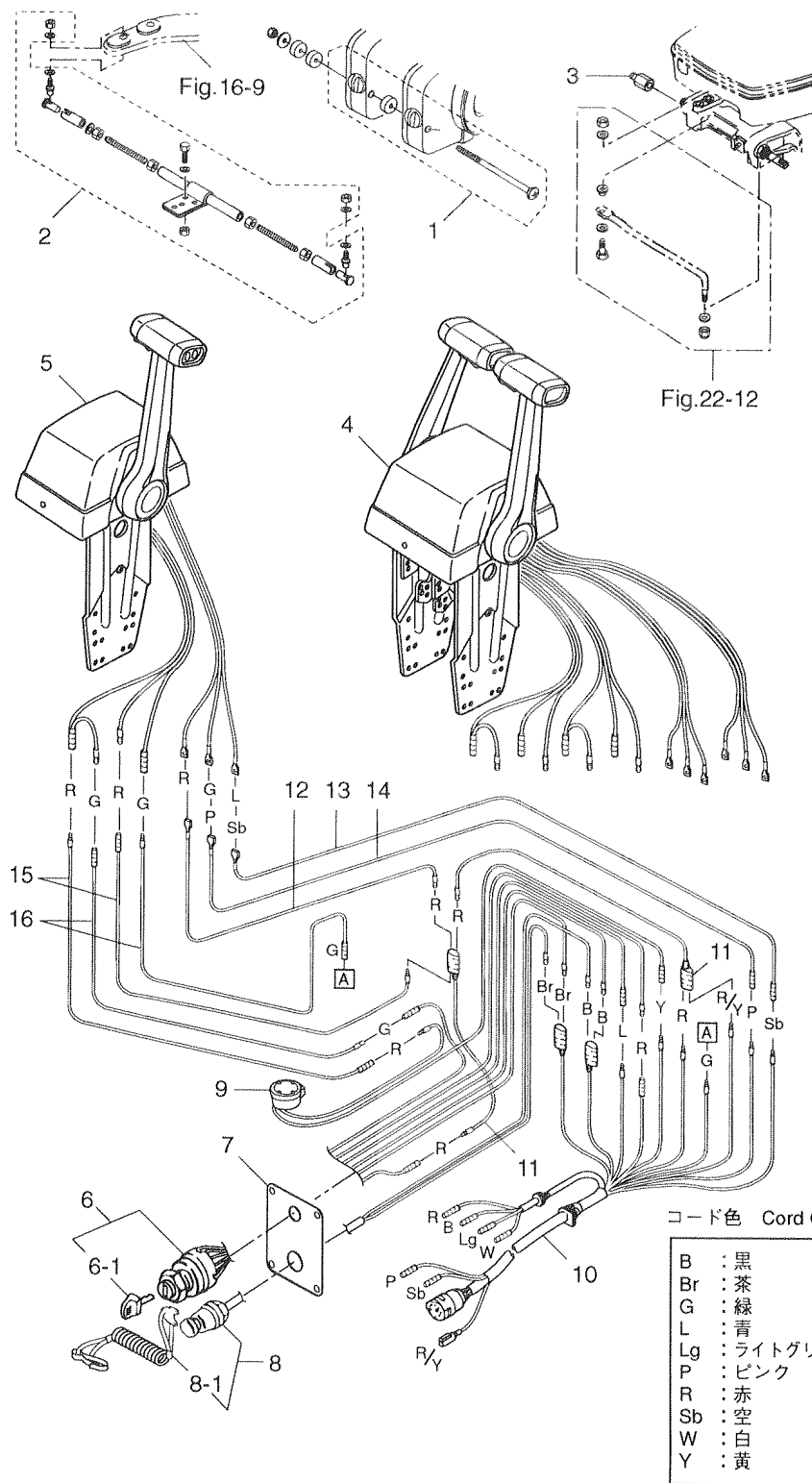
Fig. 24 OPTIONAL PARTS (2)
