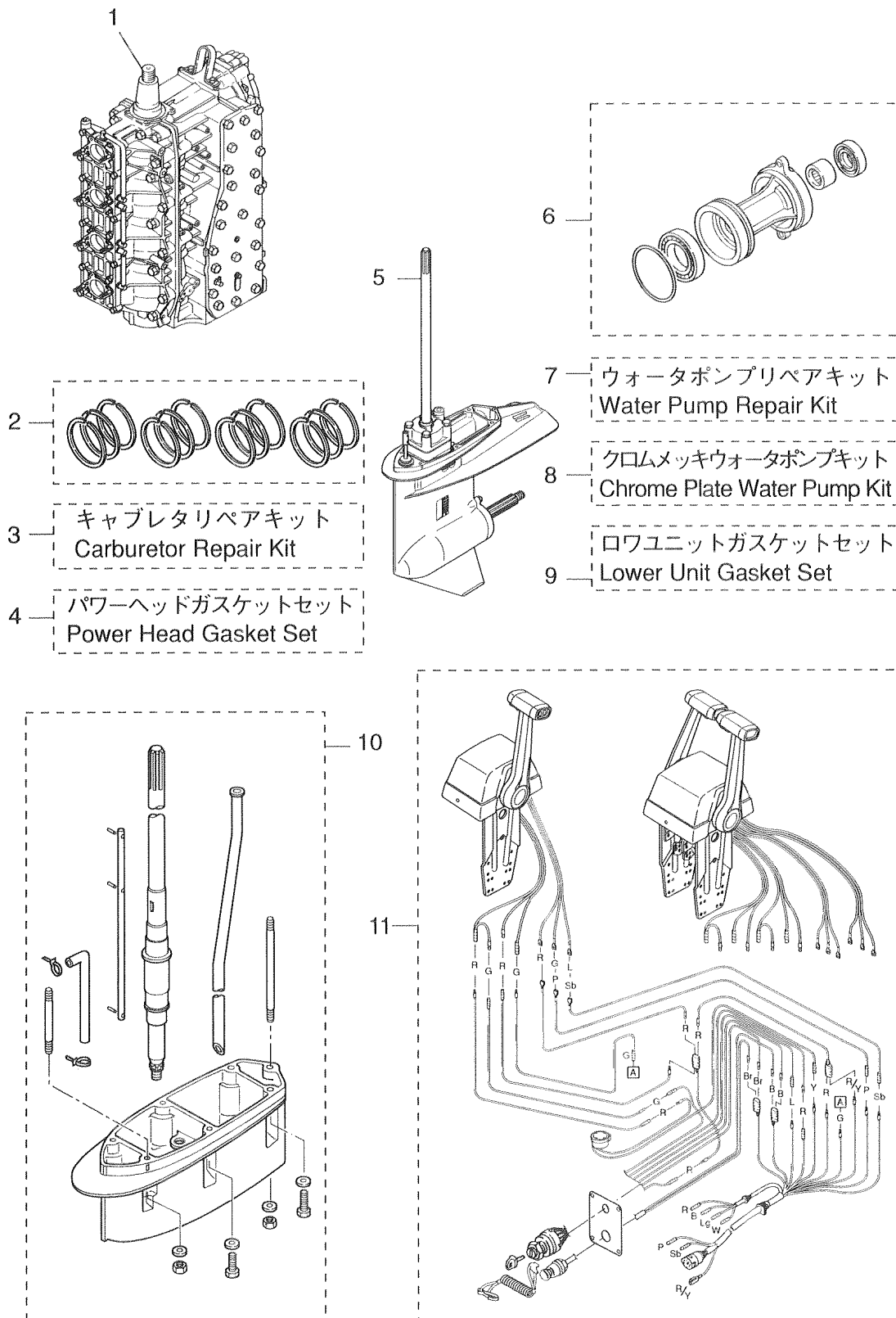
Fig. 26 ASSEMBLY · KIT
